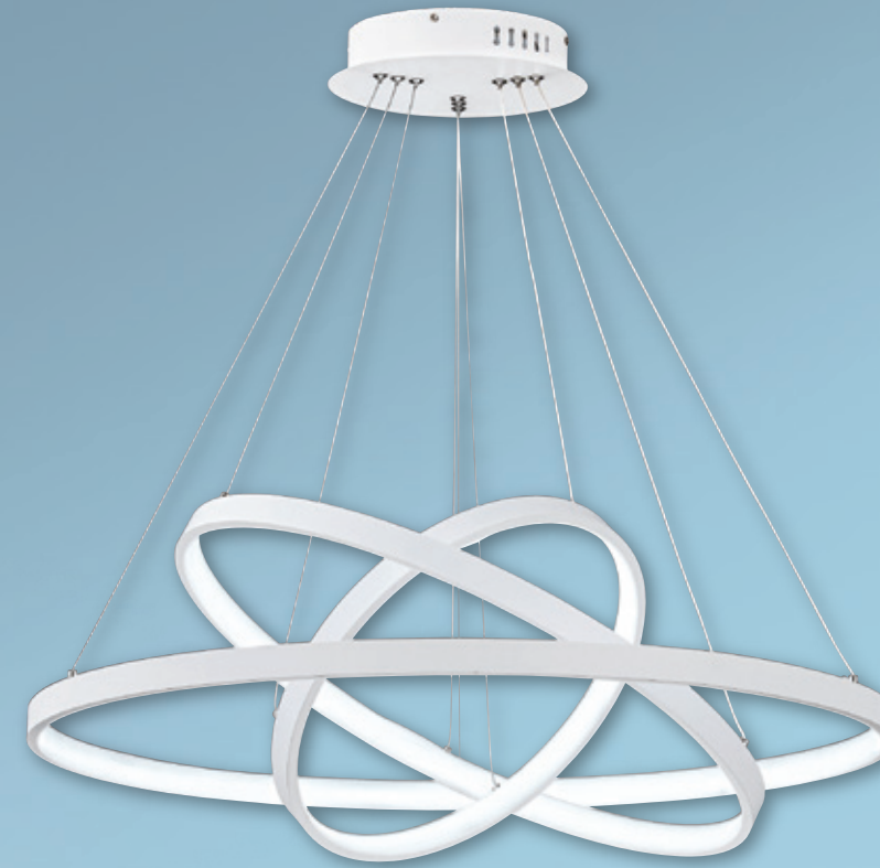
GN 70071 ( 120000 ) 寬800mm 高30mm 線長1000mm 附LED 120w、三色變光 鋁製品、造型可自由調整
