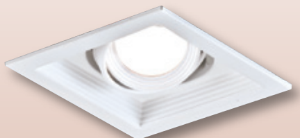
GN 7538A ( 10000 ) 長130mm 寬130mm 高120mm 附美國CREE晶片 12wx1 3000K/4000K/5700K、全電壓 防眩光
