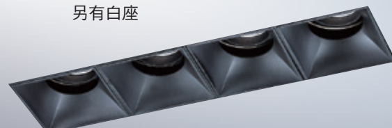
GN 7542J ( 68800 ) 長291mm 寬75mm 高105mm 附COB LED 12wx4 110v-220v、3000K/4000K/6500K 360度調角度、無邊框請準確開孔
