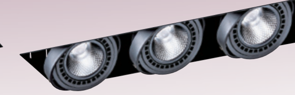
GN 7541F ( 30000 ) 長460mm 寬160mm 高90mm 附歐司朗晶片 COB 15wx3 3000K/4000K/6000K 金屬烤漆、無邊框請準確開孔
