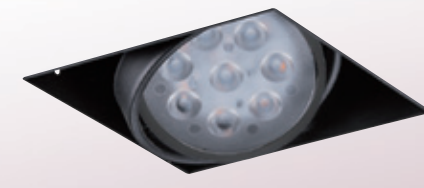
GN 75411 ( 8000 ) 長114mm 寬114mm 高90mm 附歐司朗晶片 8珠 12wx1 3000K/4000K/6000K 金屬烤漆、無邊框請準確開孔
