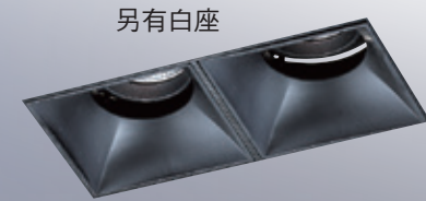
GN 7542H ( 34400 ) 長147mm 寬75mm 高105mm 附COB LED 12wx2 110v-220v、3000K/4000K/6500K 360度調角度、無邊框請準確開孔
