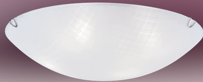
GN 73447 ( 17500 ) 寬500mm 高130mm E27x5 LED 另計 小夜燈5wx1、附電子開關 金屬烤漆、玻璃
