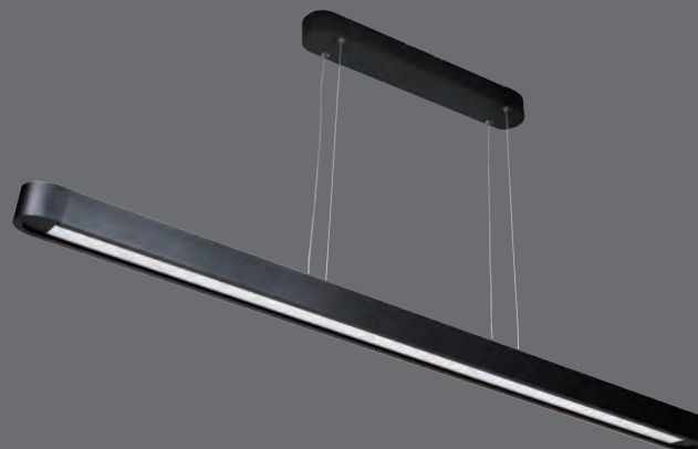
K-171-4 13000 L1260 W75 H50mm T8 x 1 另計 線長1000
