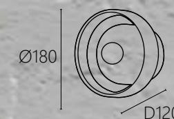
OK 20131/2 32000 Ø180 D120mm 附LED 4W x 1 3000K 大理石
