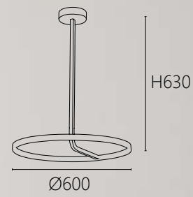
OK 21921 38000 Ø600 H630mm 內含LED 30W 4000K 鋼材烤漆 壓克力
