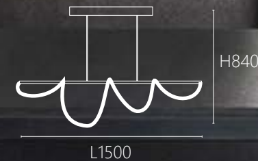
OK 21112 120000 L1500 H840mm 附LED 65W 4000K 編織硅膠 鋼材 內附明緯變壓器
