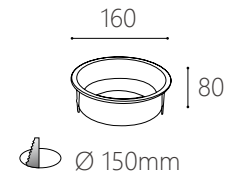
JBR 20841 材質：鋁材 尺寸：Ø160 H80 mm 嵌入孔：Ø150 mm
