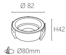
JBR 20801 材質：鋁材 尺寸：Ø82 H42 mm 嵌孔：Ø80 mm (可適用 MR16)
