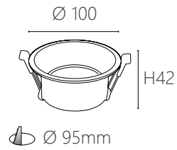
JBR 20821 L 材質：鋁材 尺寸：Ø100 H42 mm 嵌入孔：Ø95 mm (可適用 MR16)
