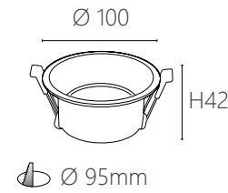
JBR 20822 L 材質：鋁材 尺寸：Ø100 H42 mm 嵌入孔：Ø95 mm (可適用 MR16)
