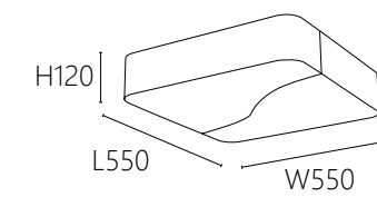
OK 21971 48000 W550 H120mm 附LED 50W 3段光色 鋼材烤漆 壓克力
