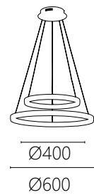
OK 21121 92000 Ø600+Ø400mm 線長2000mm 附LED 60W 3000K 皮革 鋁材
