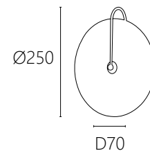
OK 20162 33000 Ø250 D70mm 內附LED 6W 3000K 雲石 鋼材
