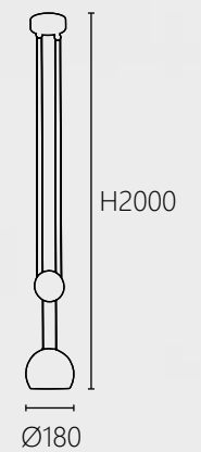
OK 21671/2 48000 Ø180 H2000mm 內附LED 5W x 1 3000K 鋼材電鍍 玻璃
