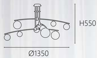
OK 20681 60000 Ø1350 H550mm G9 x 9另計 鋼材電鍍 玻璃
