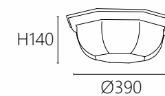
OK 20892 50000 Ø390 H140mm E27 x 3另計 全銅 玻璃
