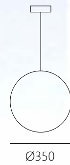
OK 21582 30000 Ø350mm 線長1500mm E27 x 1另計 鋼材 滾塑
