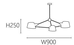
OK 20501 55000 W900 H250mm 線長1000mm E27 x 3另計 鋼材烤漆
