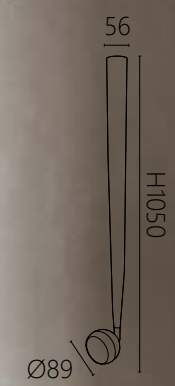
OK 21951 36000 H1050 Ø89 W56 H1050mm 內含LED 12W 3000K 鋁材 透鏡玻璃
