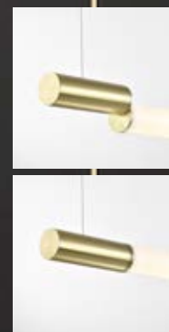
OK 21341 82000 L1300 H80mm 線長1500mm 內附LED 28W 3000K 鋁材電鍍 壓克力
