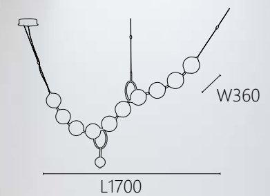
OK 21451 140000 L1700 W360mm 內含LED 5W x 10 3000K 鋼材電鍍 玻璃 內附明緯變壓器
