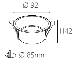
JBR 20822 M 材質：鋁材 尺寸：Ø92 H42 mm 嵌入孔：Ø85 mm (可適用 MR16)
