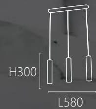
OK 21721 36000 L580 W60 H300mm 線長1000mm 內含LED 5W x 3快拆式光源 鋁材烤漆 可選3000K/4000K
