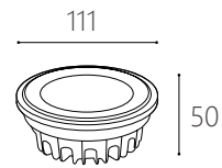
JA 12238 W 光源： PHILIPS 尺寸：Ø111 H50mm 功率：12W 通光量：1272 Lm 光色：3000K/ 4000K/ 6000K 材質：鋁材 發光角度：36° 演色性：CRI>90
