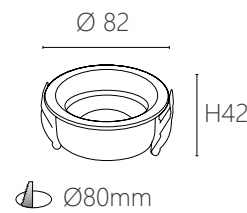
JBR 20802 材質：鋁材 尺寸：Ø82 H42 mm 嵌孔：Ø80 mm (可適用 MR16)
