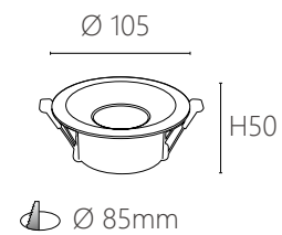
JBR 20803 材質：鋁材 尺寸：Ø105 H50 mm 嵌孔：Ø85 mm (可適用 MR16)
