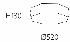
OK 20881 56000 Ø520 H130mm E27 x 4另計 全銅 玻璃
