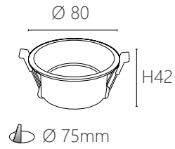
JBR 20821 S 材質：鋁材 尺寸：Ø80 H42 mm 嵌入孔：Ø75 mm (可適用 MR16)
