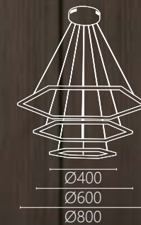
OK 21071 120000 Ø400 x 1/ Ø600 x 1/ Ø800 x 1 線長1500mm 內含LED 55W 4000K 不銹鋼電鍍 壓克力
