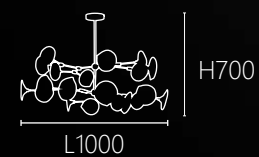
OK 20361 157000 L1000 W1000 H700mm G4 x 20另計 鋼材電鍍 玻璃 桿長300mm
