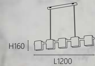
OK 20651 55000 L1200 W120 H160mm 桿長300+300mm G9 x 5另計 鋼材 玻璃
