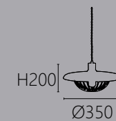
OK 21852 30000 Ø350 H200mm 線長1000mm E27 x 1 另計 鋼材烤漆
