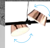
OK 20531 66000 L750 W360 H120mm 線長1500mm 附LED 8W x 4 3000K 鋼材
