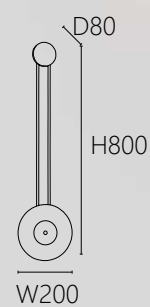
OK 20141 52000 W200 H800 D80mm 內附LED 6W 3000K 水晶砂玻璃 鋼材
