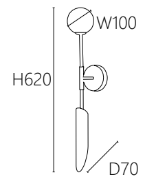
OK 20172 28000 W100 H620 D120mm G9 x 2另計 鋼材
