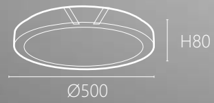
OK 22061~3 21000 Ø500 H80mm 附LED 45W 三段式光色 鋼材烤漆 壓克力
