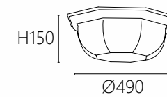
OK 20891 75000 Ø490 H150mm E27 x 4另計 全銅 玻璃
