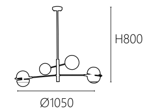
OK 20331 72000 Ø1050 H800mm G9 x 4另計/E14 x 2另計 鋼材電鍍 玻璃 桿長250+250mm
