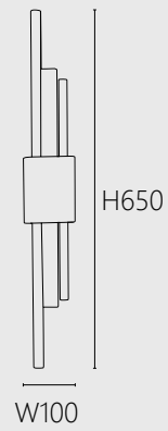
OK 20021 38000 W100 H650mm 內附LED 3W x2 3000K 大理石 鋼材
