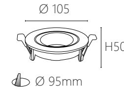
JBR 20813 材質：鋁材 尺寸：Ø105 H50 mm 嵌孔：Ø95 mm (可適用 MR16)
