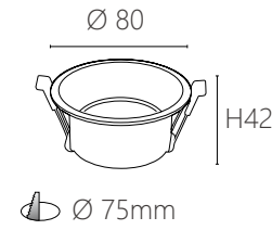
JBR 20822 S 材質：鋁材 尺寸：Ø80 H42 mm 嵌入孔：Ø75 mm (可適用 MR16)
