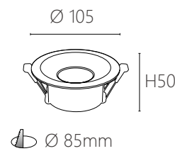
JBR 20804 材質：鋁材 尺寸：Ø105 H50 mm 嵌孔：Ø85 mm (可適用 MR16)
