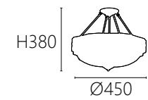
OK 20912 60000 Ø450 H380mm E27 x 4 另計 全銅 玻璃 水晶
