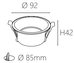
JBR 20821 M 材質：鋁材 尺寸：Ø92 H42 mm 嵌入孔：Ø85 mm (可適用 MR16)
