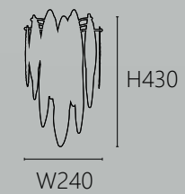
OK 21232 36000 W240 H430 D180mm E14 x 1 另計 鋼材電鍍 不銹鋼 玻璃
