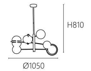
OK 20332 92000 Ø1050 H810mm G9 x 6另計/E14 x 3另計 鋼材電鍍 玻璃 桿長250+250mm
