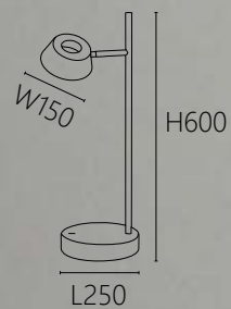
OK 20522 40000 W150 L250 H600mm 線長1500mm 附LED 8W x 1 3000K 鋼材 附開關
