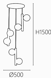
OK 21301 90000 Ø500 H1500mm G9 x 6 另計 鋼材烤漆 玻璃 線長1500mm
