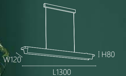
OK 21351 96000 L1300 W120 H80mm 線長1500mm 內附LED 36W 全電壓 3000K 鋁材 實木
