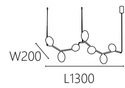
OK 20481 95000 L1300 W200mm 線長1000mm G9 x 7另計 玻璃 鋼材烤漆
