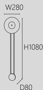
OK 20142 60000 W280 H1080 D80mm 內附LED 6W 3000K 水晶砂玻璃 鋼材
