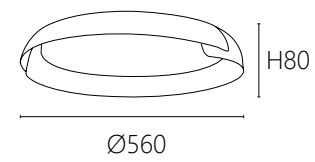
OK 21981/2 38000 Ø560 H80mm 附LED 36W x 2 3段光色 鋼材烤漆 壓克力
