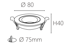
JBR 20812 材質：鋁材 尺寸：Ø80 H40 mm 嵌孔：Ø75 mm (可適用 MR16)
