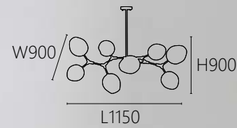
OK 20401 90000 L1150 W900 H900mm E27 x 8另計 鋼材烤漆 玻璃 桿長250+250mm
