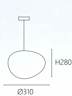
OK 21581 24000 Ø310 H280mm 線長1500mm E27 x 1另計 鋼材 滾塑
