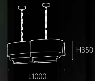
OK 20751 320000 L1000 W320 H350mm 鏈長1000mm E14 x 12 另計 鋼材 手工玻璃
