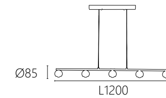
OK 20631 90000 L1200 Ø85mm 線長1500mm 內附LED 5W x 5 3000K 鋁材 透鏡玻璃
