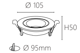
JBR 20814 材質：鋁材 尺寸：Ø105 H50 mm 嵌孔：Ø95 mm (可適用 MR16)
