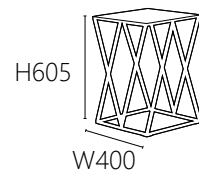
OK 21022 160000 L400 W400 H605mm 附LED 64W 4000K 不銹鋼電鍍 壓克力
