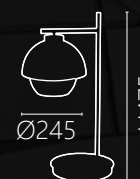
OK 20963 38000 Ø245 H475mm E27 x 1 另計 鋼材烤漆 玻璃
