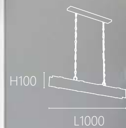
OK 20561 78000 L1000 W75 H100mm 鏈長600mm 內含LED 5W x 4快拆式光源 實木 鋼材 可選3000K/4000K
