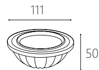
JA 1662 B 光源： PHILIPS 尺寸：Ø111 H50mm 功率：16W 通光量：1696 Lm 光色：3000K/ 4000K/ 6000K 材質：壓鑄鋁 發光角度：24° 演色性：CRI>90
