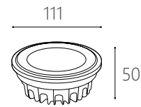
JA 12238 B 光源： PHILIPS 尺寸：Ø111 H50mm 功率：12W 通光量：1272 Lm 光色：3000K/ 4000K/ 6000K 材質：鋁材 發光角度：36° 演色性：CRI>90
