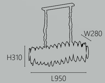
OK 21231 168000 L950 W280 H310mm 鏈長600mm E14 x 6 另計 鋼材電鍍 不銹鋼 玻璃
