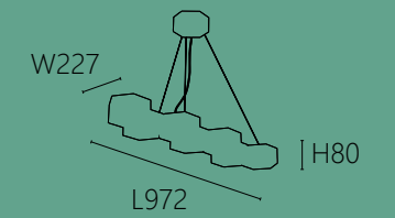
OK 20872 52000 L972 W227 H80mm 線長1000mm 內附LED 7W x 4 木材 可選3000K/4000K
