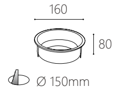
JBR 20842 材質：鋁材 尺寸：Ø160 H80 mm 嵌入孔：Ø150 mm
