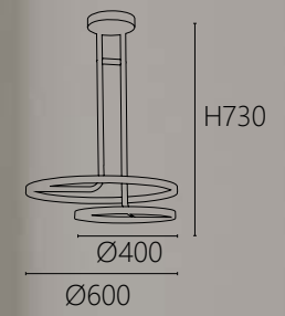
OK 21931 72000 Ø400+Ø600 H730mm 內含LED 45W 4000K 鋼材烤漆 壓克力
