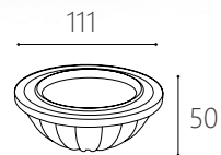
JA 1662 W 光源： PHILIPS 尺寸：Ø111 H50mm 功率：16W 通光量：1696 Lm 光色：3000K/ 4000K/ 6000K 材質：壓鑄鋁 發光角度：24° 演色性：CRI>90
