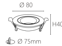
JBR 20811 材質：鋁材 尺寸：Ø80 H40 mm 嵌孔：Ø75 mm (可適用 MR16)
