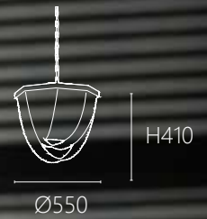
OK 21191 250000 Ø550 H410mm 鏈長800mm E14 x 11另計 鋼材電鍍 水晶串珠
