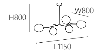
OK 20411 60000 L1150 W800 H800mm E27 x 5另計 鋼材烤漆 玻璃 桿長250+250mm
