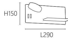
OK 20082 26000 L290 D110 H150mm 內含LED 5W 3000K 鋼材烤漆 可無線充電
