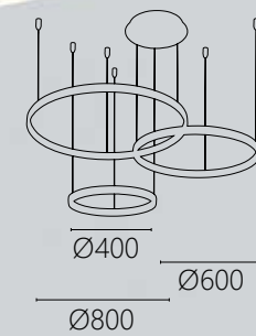
OK 21131 140000 Ø800+Ø600+Ø400mm 線長1200mm 附LED 108W 3000K 皮革 鋁材
