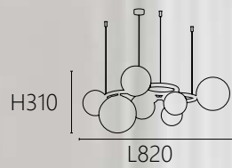
OK 20421 88000 L820 W705 H310mm 線長1500mm G9 x 7 另計 鋼材 煙灰色玻璃
