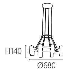
OK 21441 132000 Ø680 H140mm 線長1000mm 內含LED 5W x 8 快拆式光源 鋁材電鍍 可選3000K/4000K
