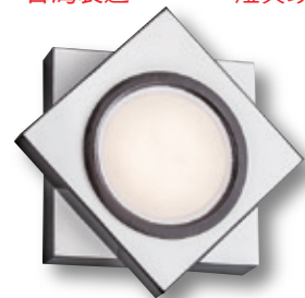
GN 7476H ( 16300 ) 寬250mm 高250mm 深70mm 附LED 14wx1、3000K/4000K/5700K 鋁製品、金屬、擴散板 燈具嵌孔120mm、台灣製造
