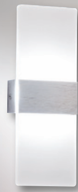
GN 7468J ( 9500 ) 寬100mm 高270mm 深40mm 附LED 7w 鋁製品、壓克力
