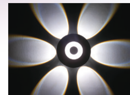
GN 74637 ( 17500 ) 寬120mm 高120mm 深65mm 附LED 2wx1、1wx6 鋁合金、(裝潢板適用)
