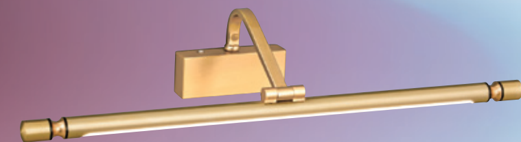
GN 74632 ( 36300 ) 寬630mm 高130mm 深200mm 附LED 12w、三段分色、白光、黃光、雙色光 鋼材、壓克力、(裝潢板適用)
