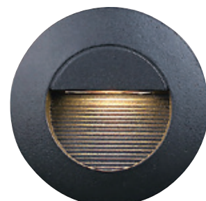
GN 7564A ( 15700 ) 寬83mm 高83mm 深55mm 附LED 1w 鋁製品、玻璃、附預埋盒 預埋盒：寬65mm 深42mm
