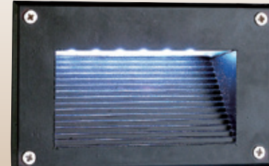
GN 7564J ( 15800 ) 寬165mm 高100mm 深65mm 附LEDx30粒 110v-220v、3000K/6500K/藍 附預埋盒：寬160mm 高100mm 深70mm、牆角燈
