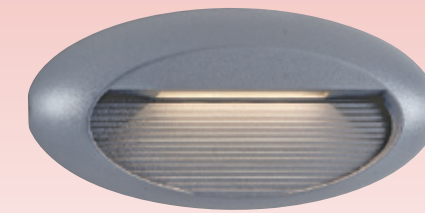
GN 75651 ( 32500 ) 寬266mm 高130mm 深55mm 附LED 5wx1 鋁製品、玻璃燈罩
