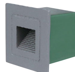
GN 7564F ( 12500 ) 寬58mm 高58mm 深55mm 附LED 1w 鋁製品、壓克力、附預埋盒 預埋盒：寬45mm 高45mm 深45mm
