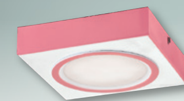
GN 7315B ( 15000 ) 長200mm 寬200mm 高40mm 附LED 16wx1 3000K/4000K/5700K 鋁製品、金屬、擴散板 燈具嵌孔150mm、 台灣製造
