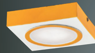
GN 73156 ( 12500 ) 長180mm 寬180mm 高40mm 附LED 14wx1 3000K/4000K/5700K 鋁製品、金屬、擴散板 燈具嵌孔120mm、 台灣製造
