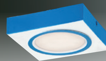
GN 73159 ( 15000 ) 長200mm 寬200mm 高40mm 附LED 16wx1 3000K/4000K/5700K 鋁製品、金屬、擴散板 燈具嵌孔150mm、 台灣製造
