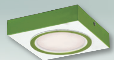
GN 7315F ( 15000 ) 長200mm 寬200mm 高40mm 附LED 16wx1 3000K/4000K/5700K 鋁製品、金屬、擴散板 燈具嵌孔150mm、 台灣製造
