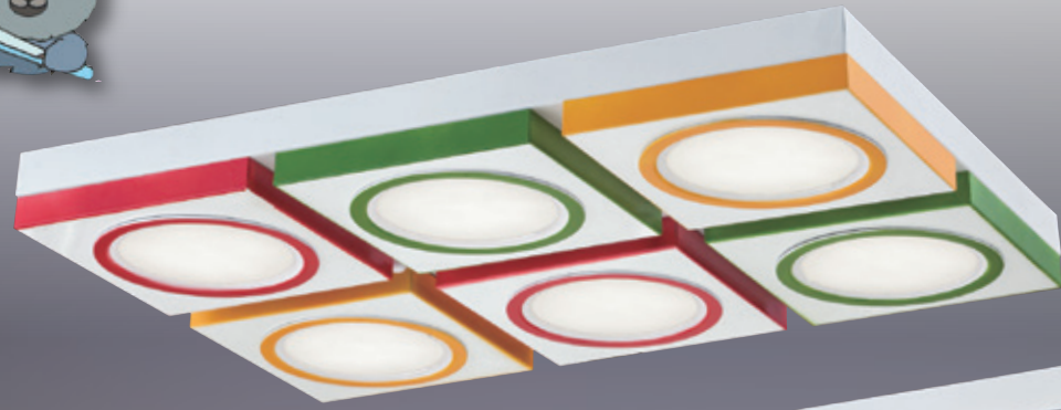
GN 73141 ( 112500 ) 長660mm 寬440mm 高70mm 附LED 16wx6 3000K/4000K/5700K 附小夜燈電子泡、附電子開關 鋼材、壓克力、 台灣製造
