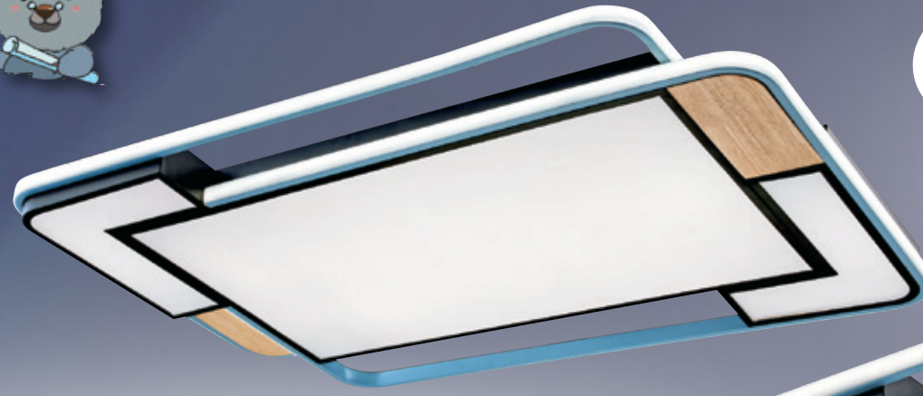
GN 73081 ( 106800 ) 長900mm 寬600mm 高50mm 附LED 100w (分段切換三色溫) 鐵材烤漆黑/藍、木製品、壓克力
