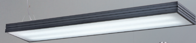
GN 74944 ( 33300 ) 長1250mm 寬250mm 高60mm 線長1000mm 附T8 LED燈管 4尺 20wx2 鋁合金烤平光黑、壓克力燈罩 可改3燈 另計
