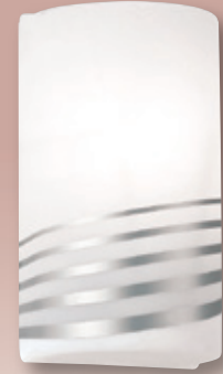
GN 7482A ( 7000 ) 寬120mm 高210mm 深80mm E27x1 LED 另計 壓克力印刷、台灣製造
