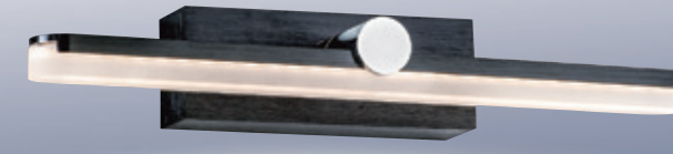
GN 74411 ( 25000 ) 寬300mm 高50mm 深90mm 附LED 7w、3000K 壓鑄鋁、壁座：寬140mm 高50mm
