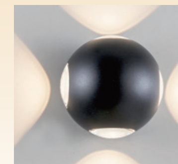
GN 7443H ( 18800 ) Ø100mm 深80mm 附LED 3wx4、3000K 鋁製品、光源四面亮 壁座：Ø65mm
