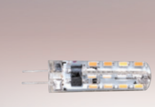
GN J23 ( 1300 ) 寬10mm 高33mm G4燈頭 LED 3.5w 110v
